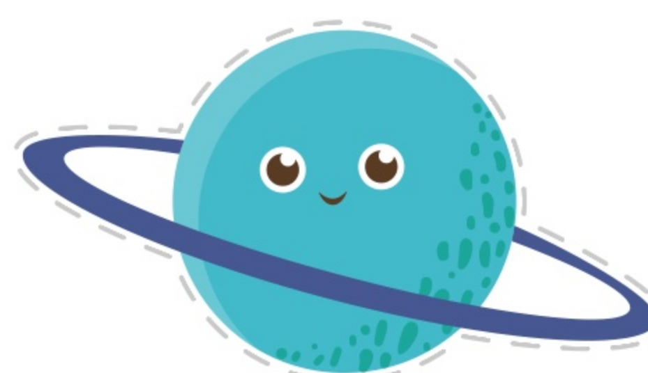
URÁN
