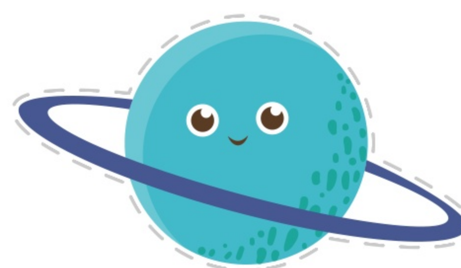
URAN
