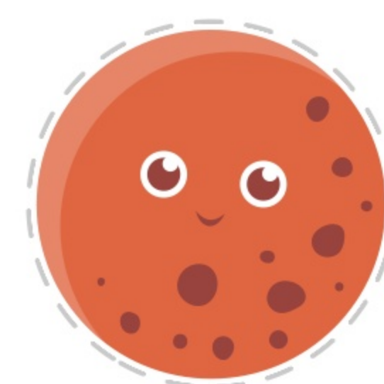
MARS
